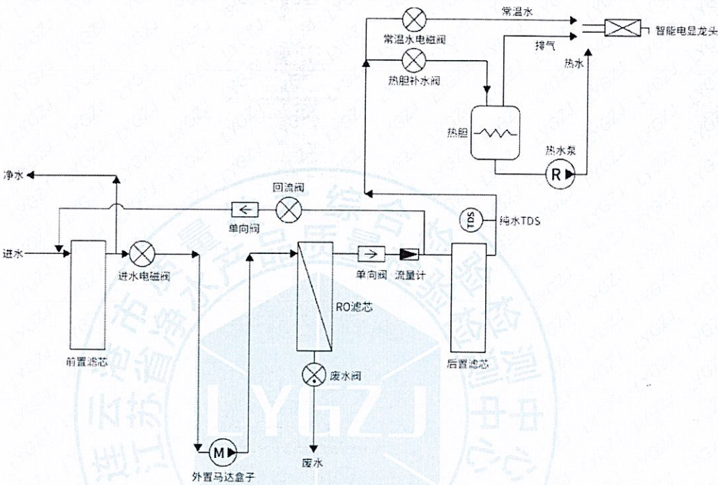
ERH-X10 (水处理工艺图)
