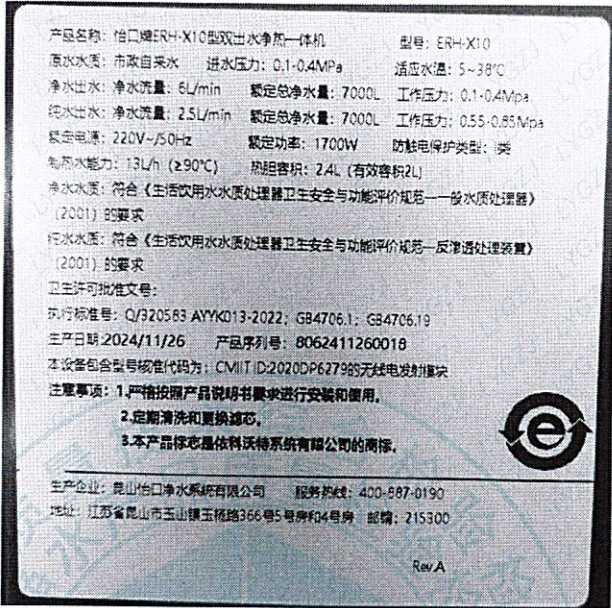
ERH-X10 (铭牌)
